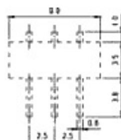
P.C.B. LAYOUT
